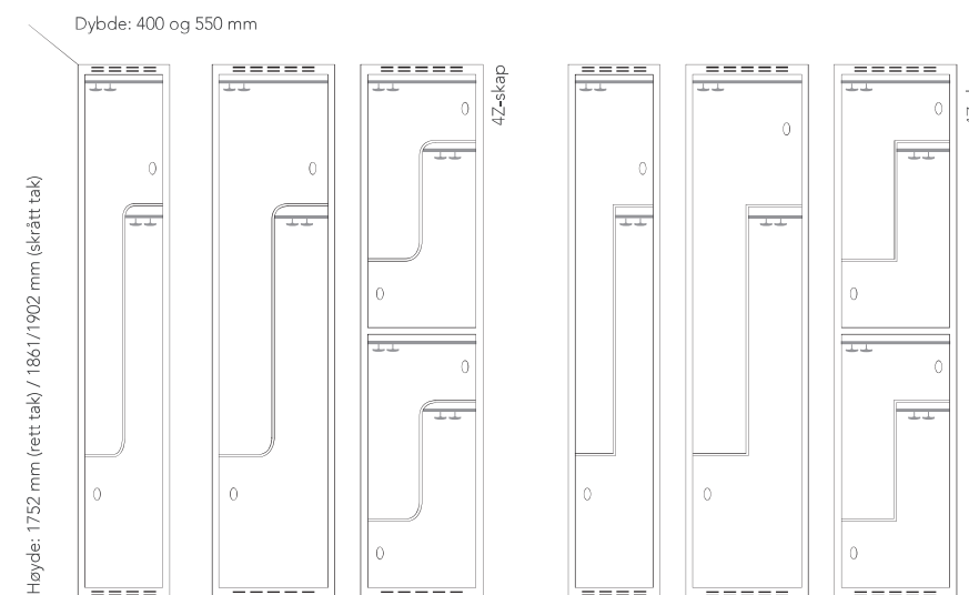
Bredde: 300 (gjelder ikke 4Z) og 400 mm. Buet laminatdør og rett ståldør
