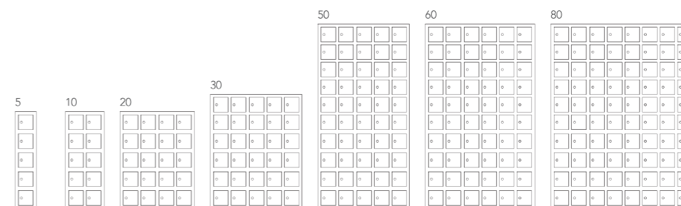
5: HxB: 780 x 210 mm. 21 kg - 10: HxB: 780 x 390 mm. 31 kg - 20: HxB: 780 x 750 mm. 58 kg - 30: HxB: 930 x 930 mm. 94 kg 50: HxB: 1530 x 930 mm. 132 kg - 60: HxB: 1530 x 1110 mm. 162 kg - 80: HxB: 1530 x 1470 mm. 211 kg
